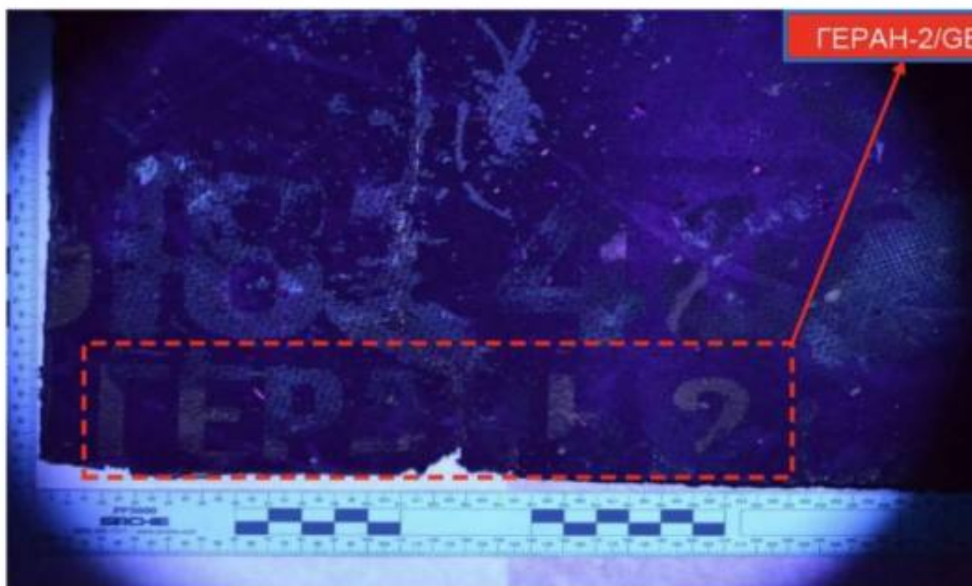
Fig. 3 – Inscripția „ГЕРАН-2/ Geran-2” prezentă la nivelul fragmentului de aeronavă
